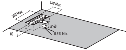
Instalación modelo Gandía Plus
